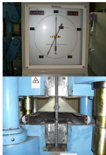
鉄筋引張試験機
